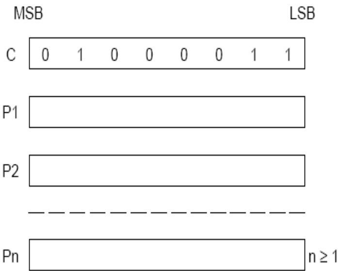
Figure 25. MREAD parameters
