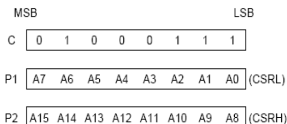
Figure 23. CSRR parameters
