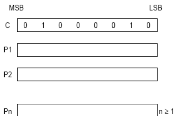
Figure 24. MWRITE parameters
