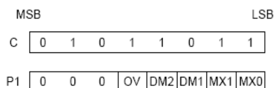
Figure 17. OVLAY parameters
