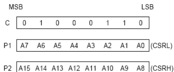
Figure 22. CSRW parameters
