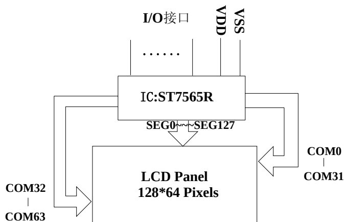
图 2:ZX12864G-139-P 图像点阵型液晶模块的电路框图
