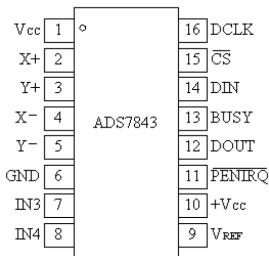
图 3 ADS7843 引脚
