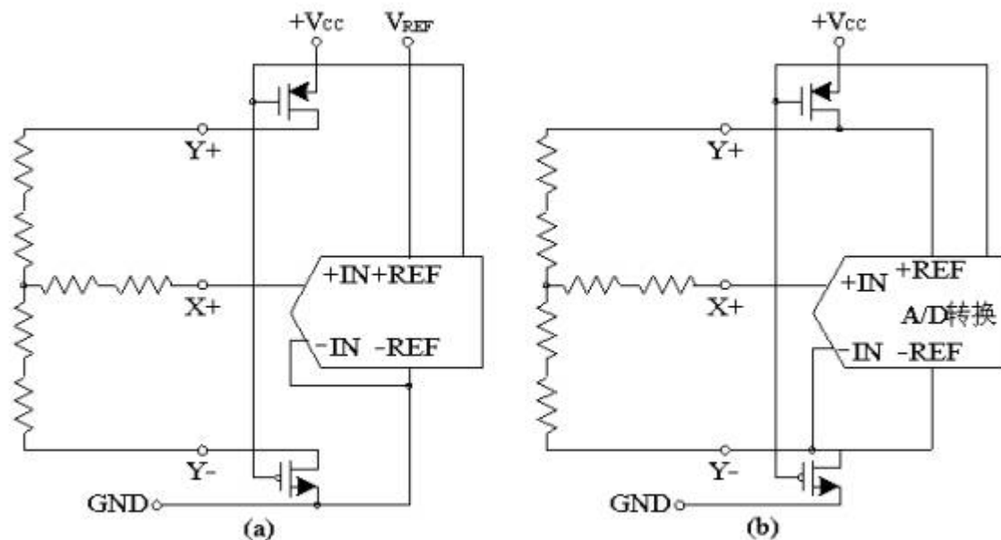
图 6 参考电压输入模式
