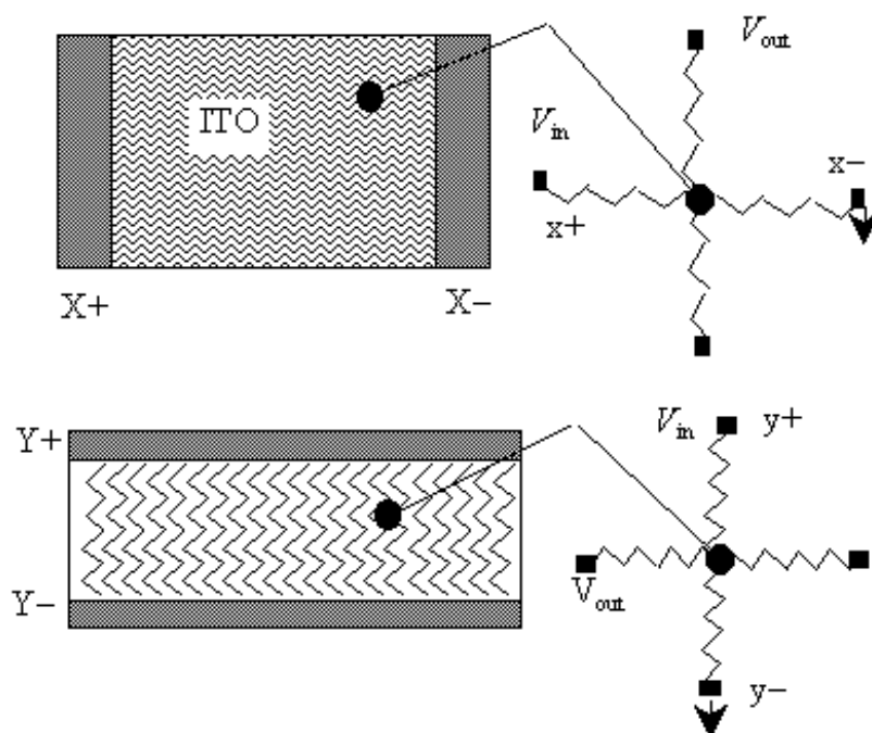
图 2 工作时的导体层
