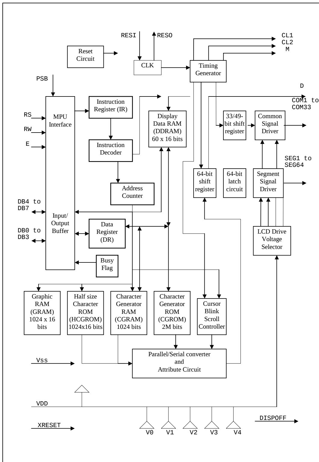
系統方塊圖
