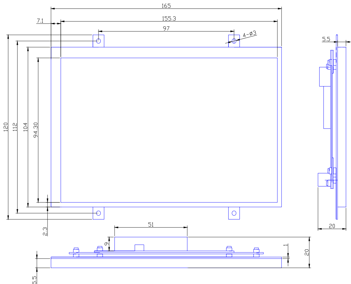
LR-070ARM液晶显示器铁板安装尺寸图
