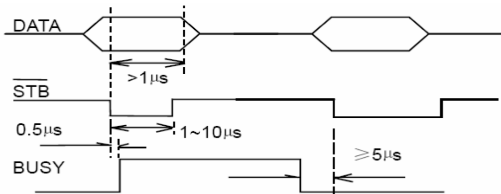
并行口时序图
