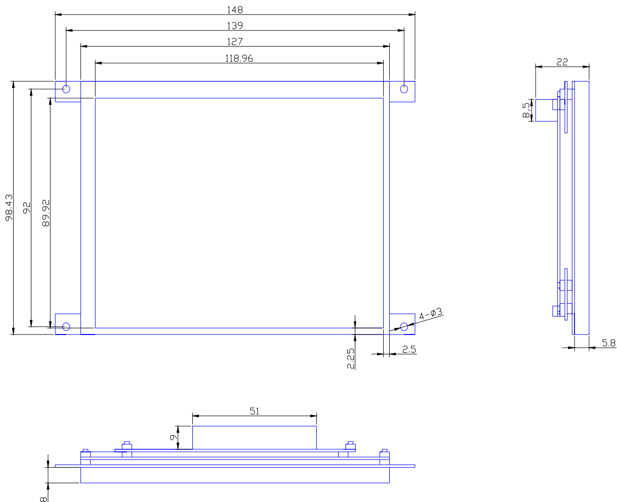
LR-057ARM液晶显示器铁板安装尺寸图
