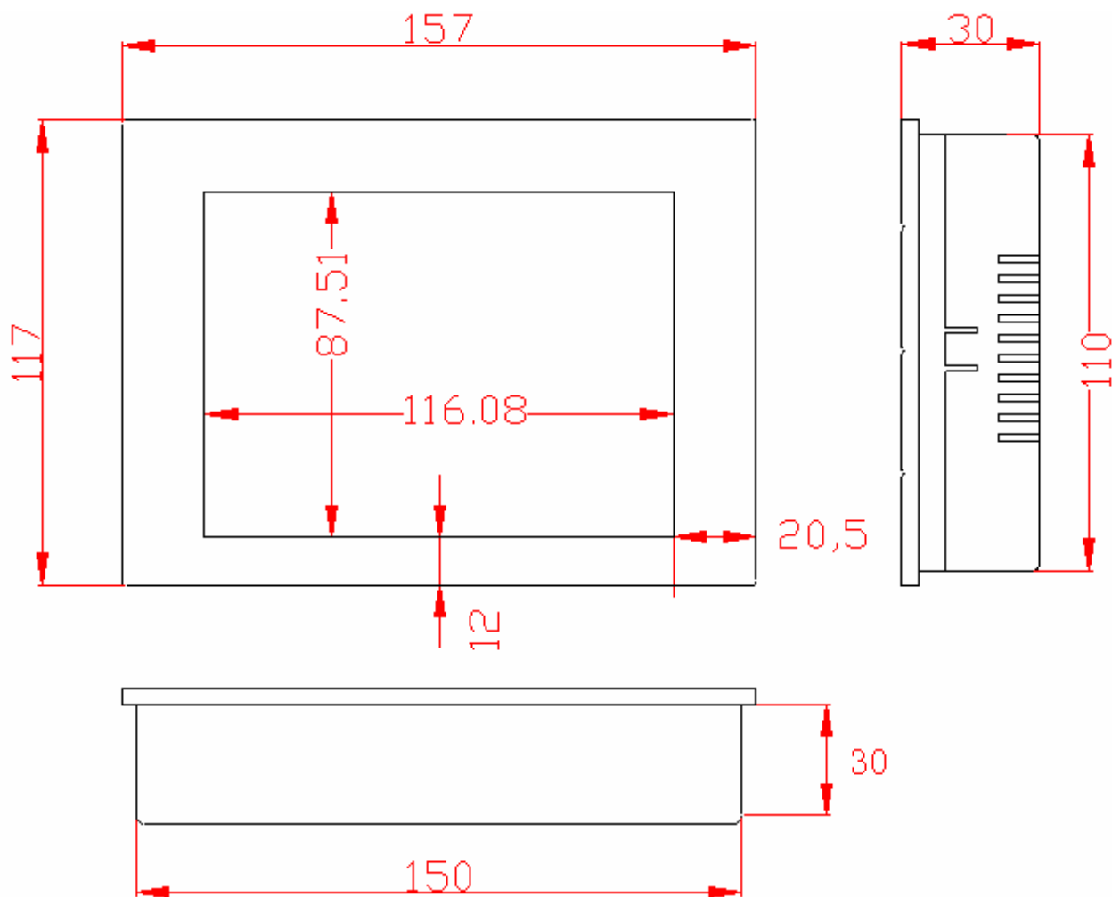
LR-056VRAM液晶显示器金属外壳安装尺寸图
