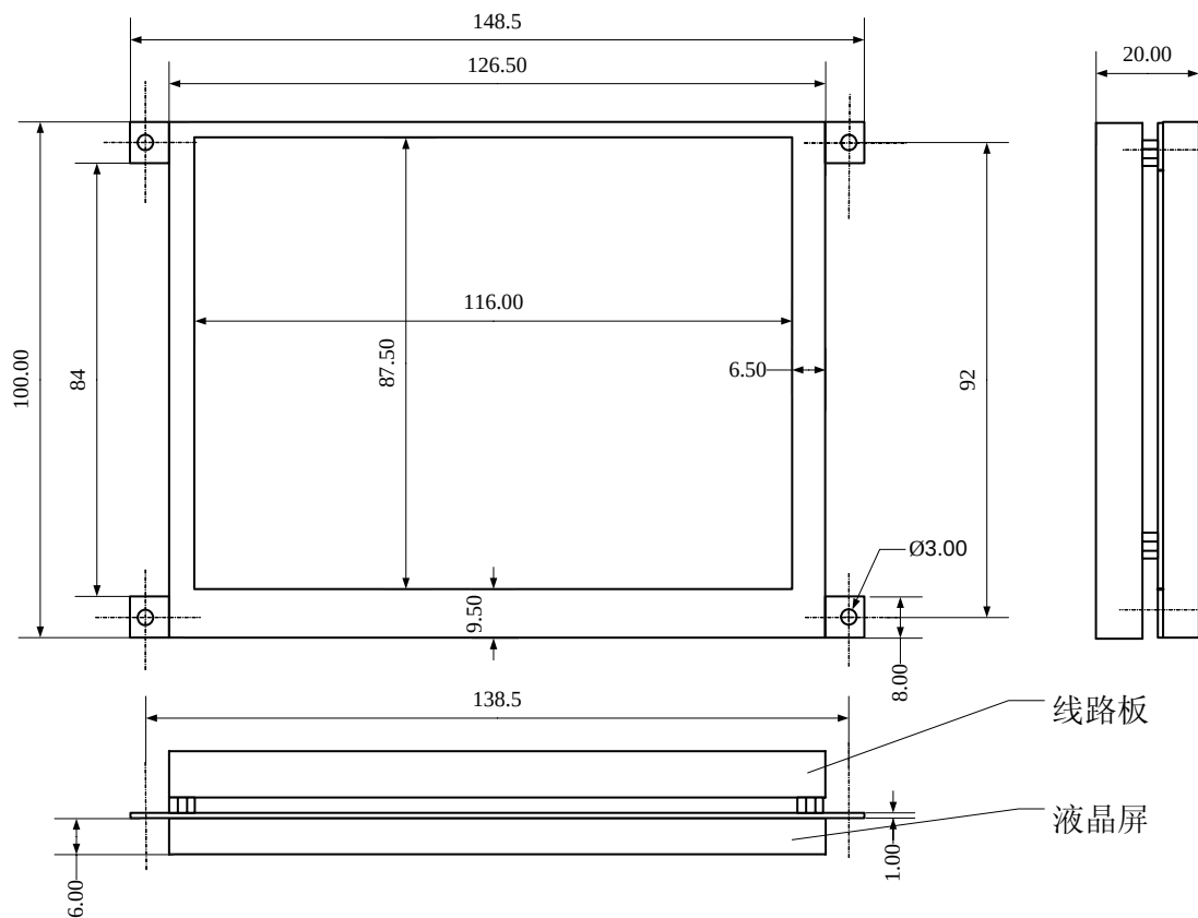
LR-056ARM液晶显示器铁板安装尺寸图
