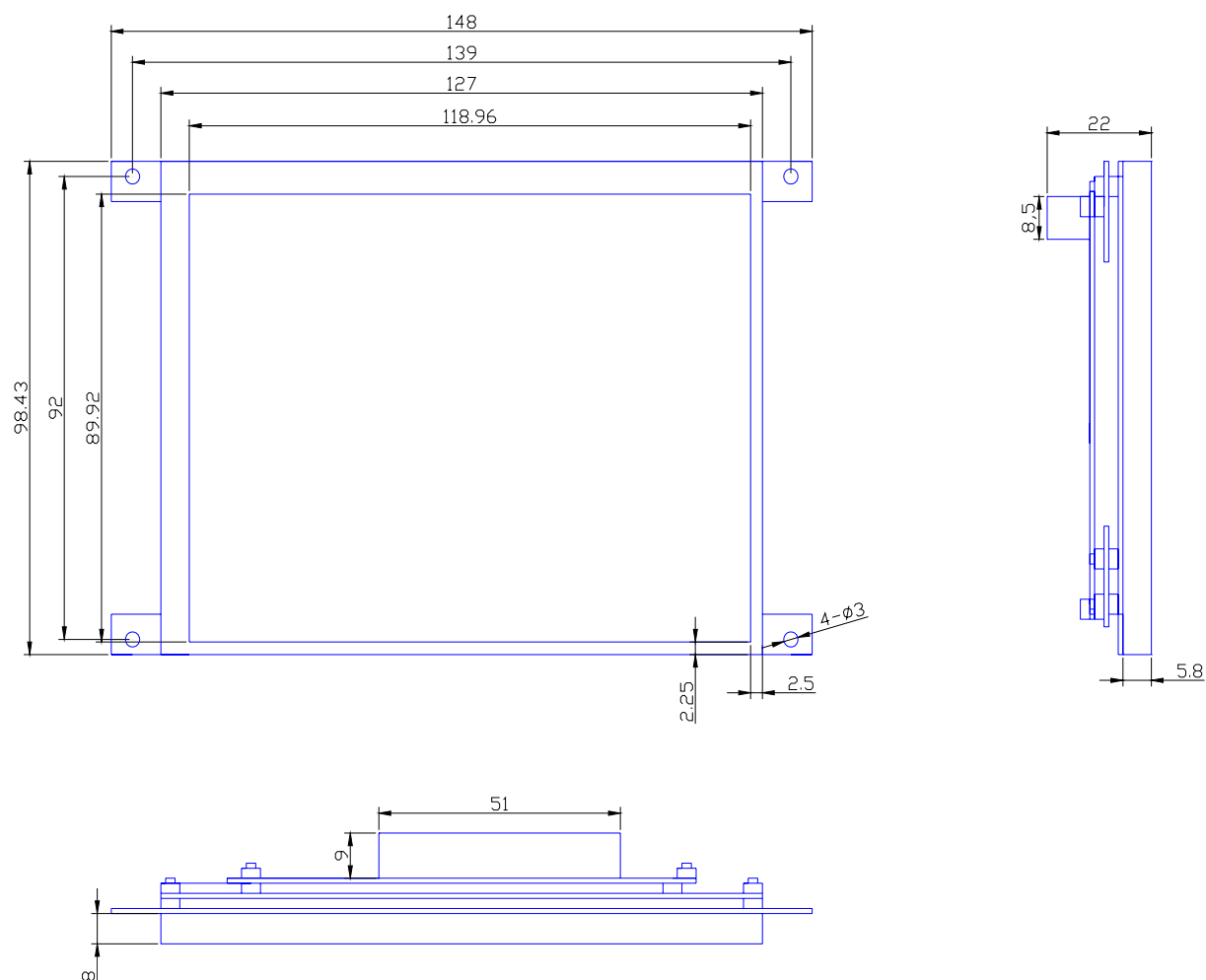
LR-057VRAM液晶显示器铁板安装尺寸图
