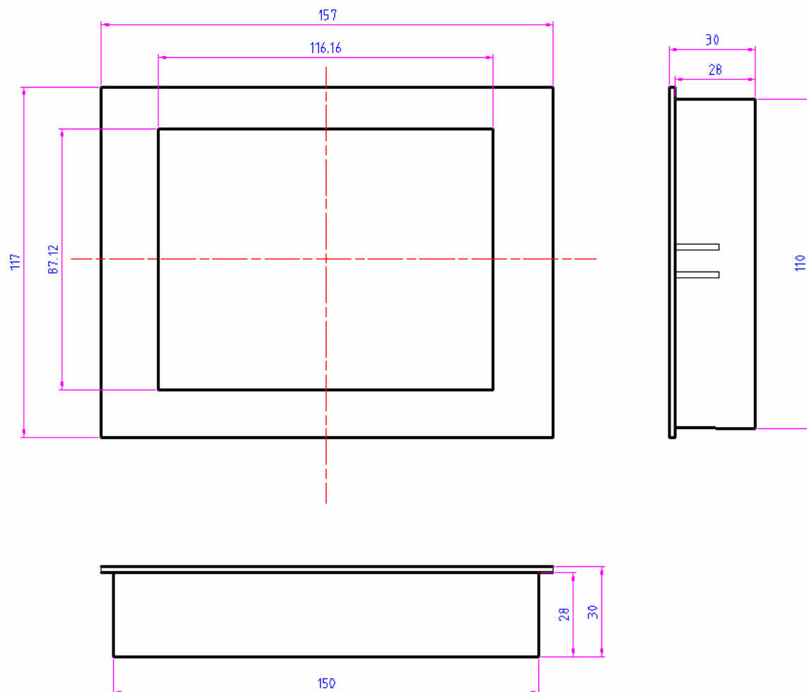
LR-057VRAM液晶显示器铁壳安装尺寸图
